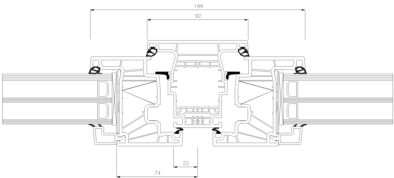
Mullion 92 PULS ARTEVO® - 1555565 Flügel Z64 PULS ARTEVO® max - 1555229
