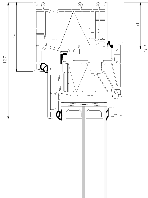
Blendrahmen 75 PULS ARTEVO® max - 1555635 Flügel Z64 PULS ARTEVO® max - 1555229
