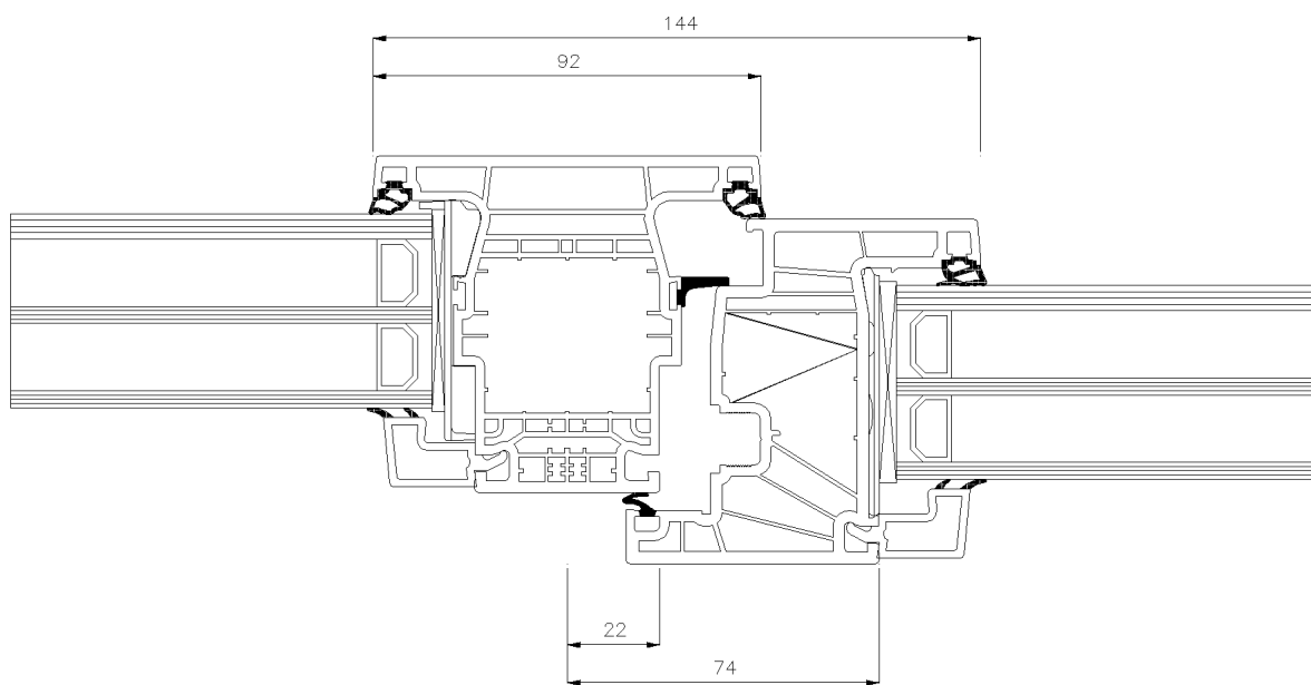
Mullion 92 PULS ARTEVO® - 1555565 Flügel Z64 PULS ARTEVO® max - 1555229
