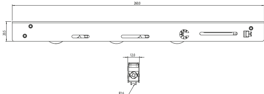
Door Roller Profile Art. No. 328672
